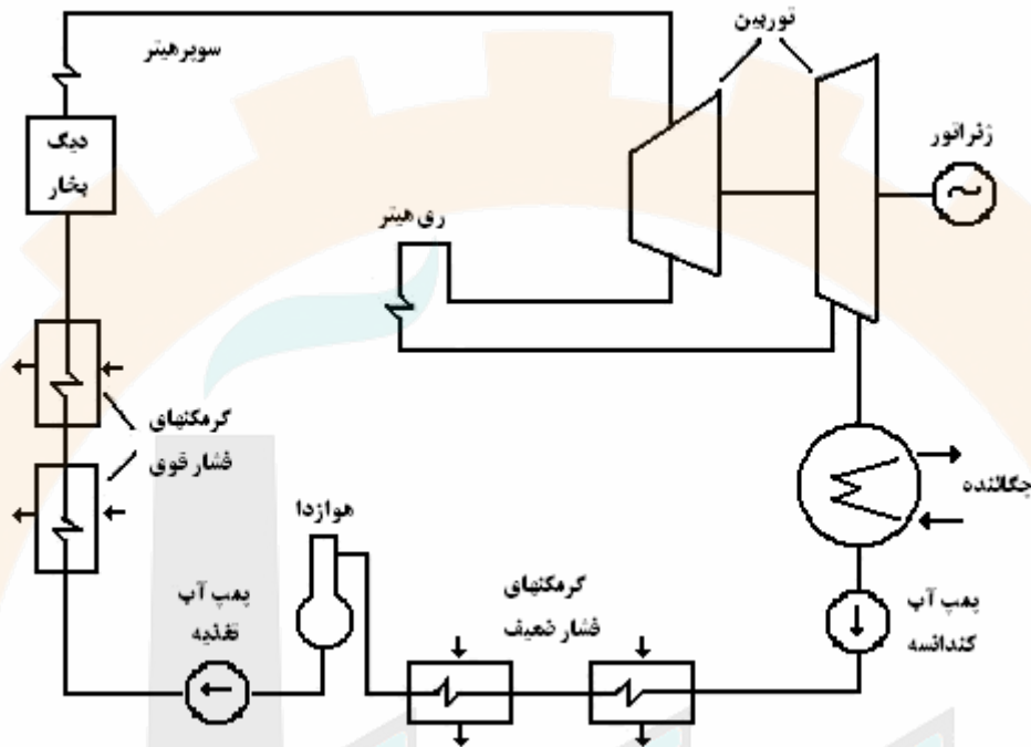
شکل ۳-۱: شماتیک چرخه آب و بخار در یک نیروگاه حرارتی بخار
