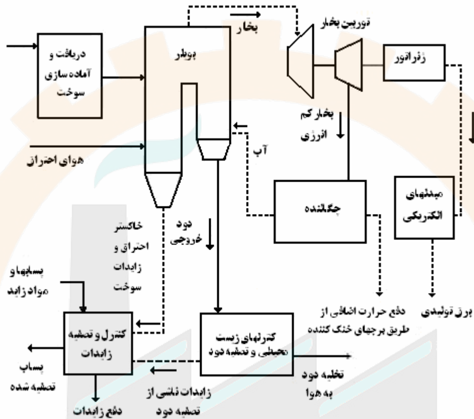
شکل ۱-۲: اجزای اساسی یک نیروگاه حرارتی با توربین بخار
