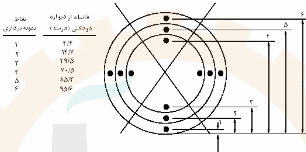
شکل ۶-۷: نحوه جانمایی نقاط اندازه گیری در دودکشا
