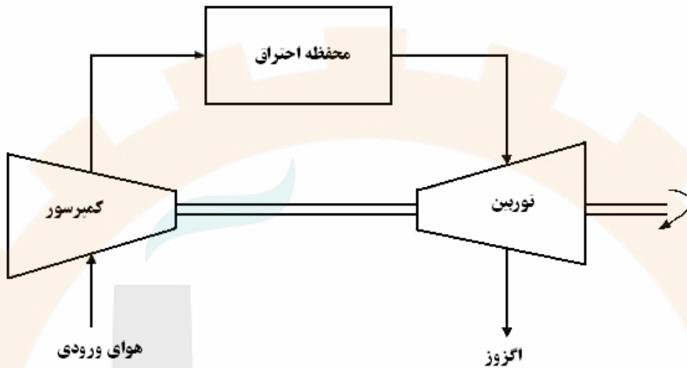
شکل ۵-۱: شماتیک یک چرخه مستقیم توربین گازی
